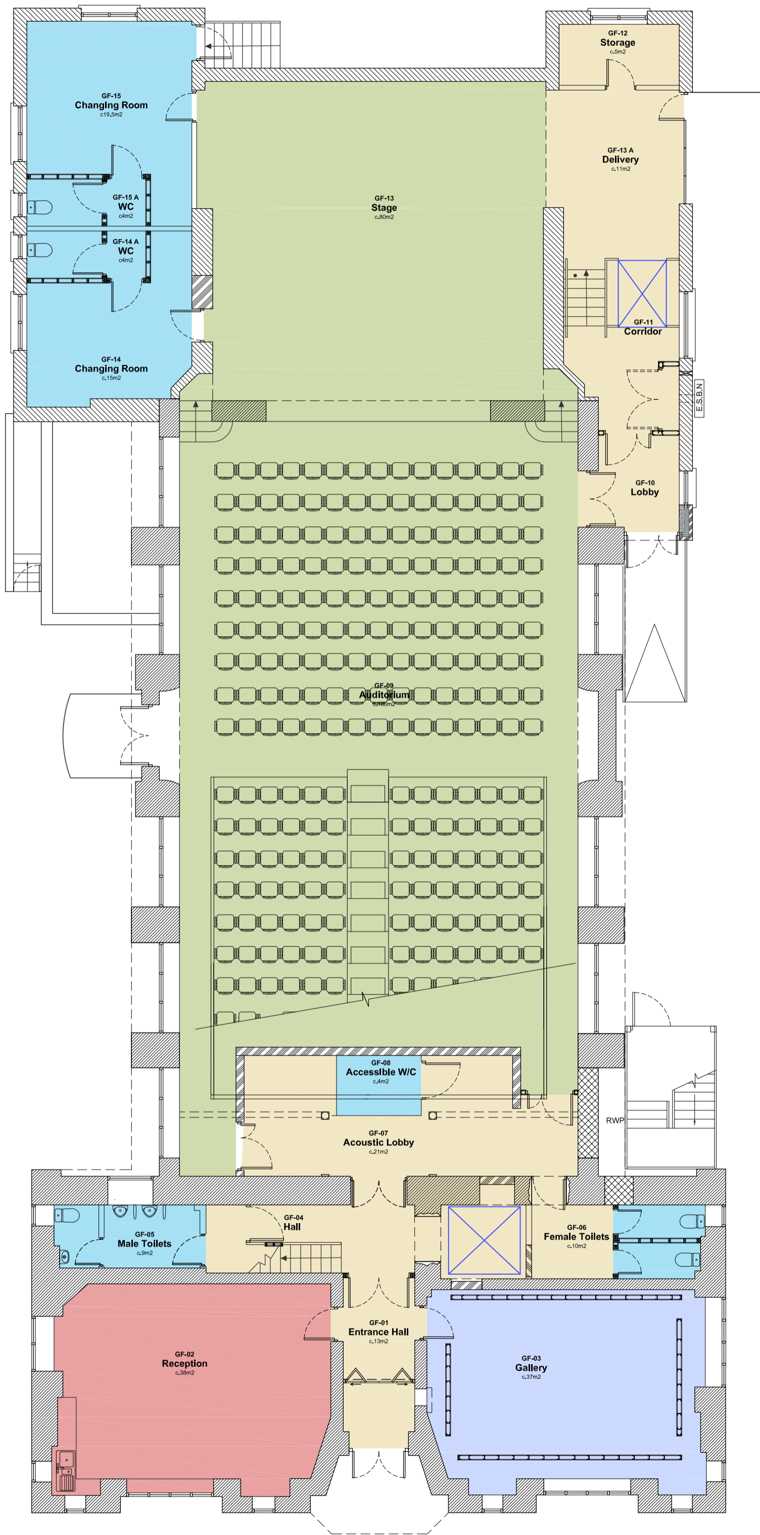
G r o u n d F l o o r P l a n
